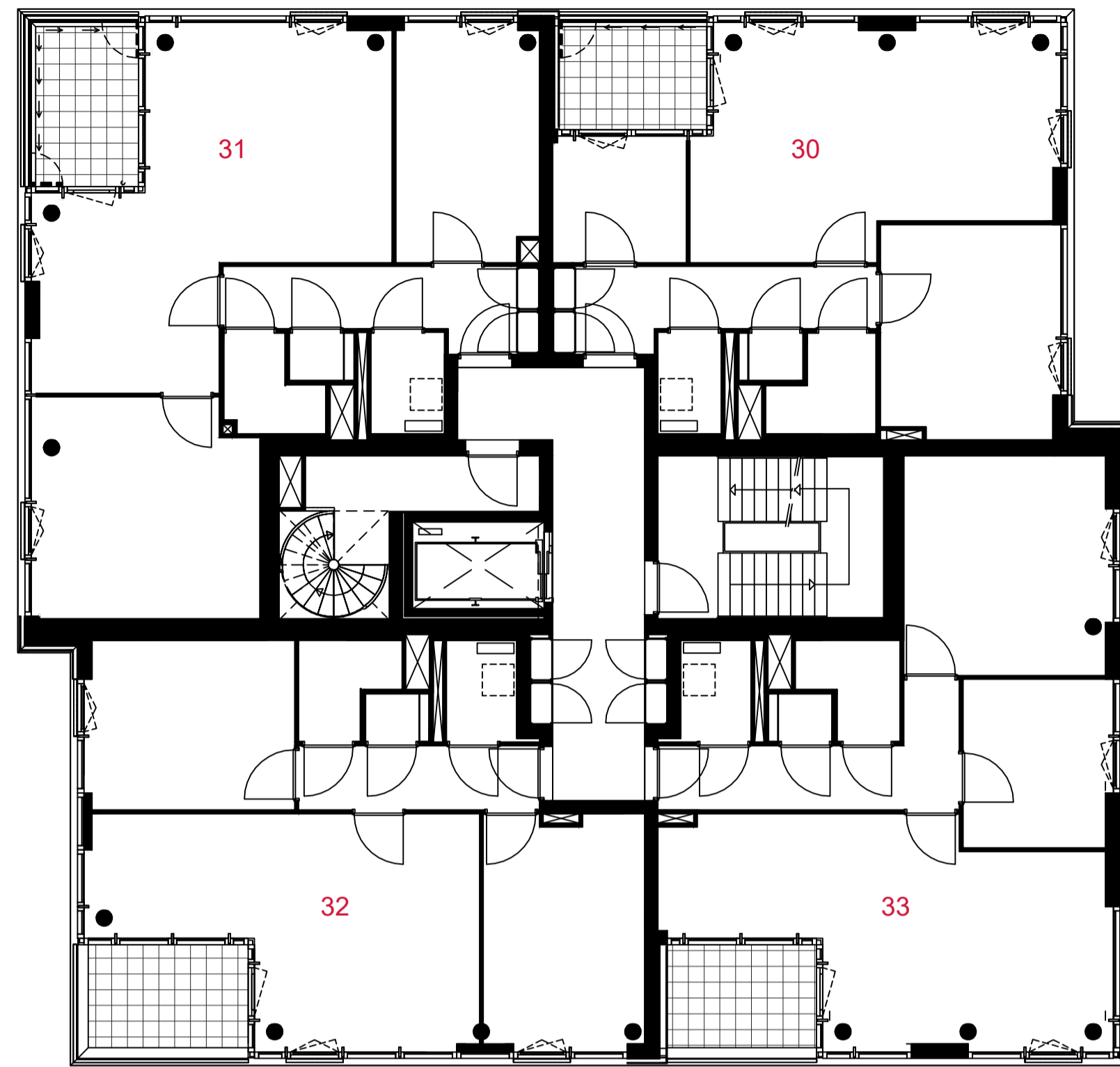
2e verdieping
