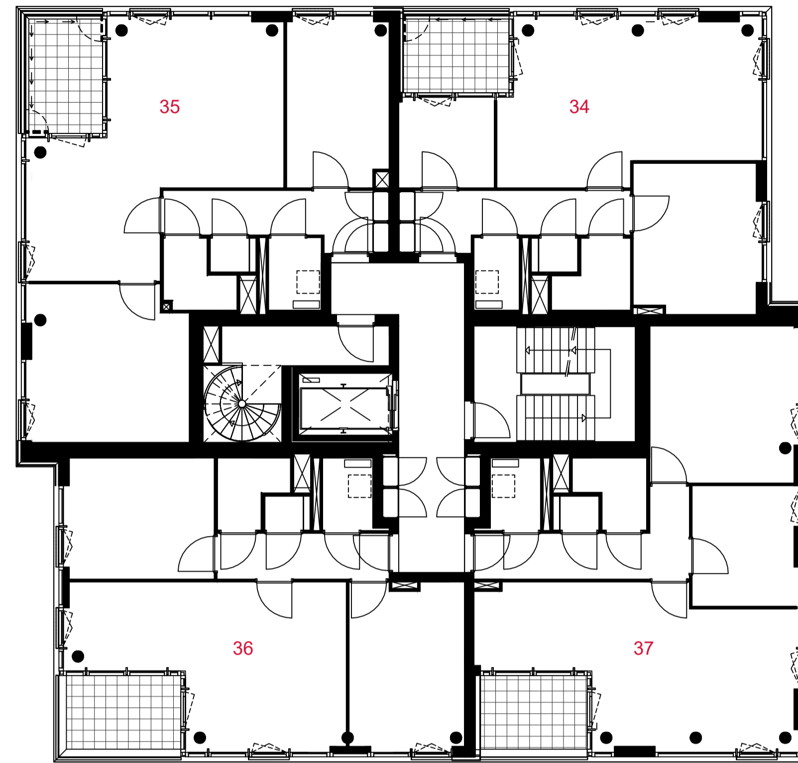
3e verdieping
